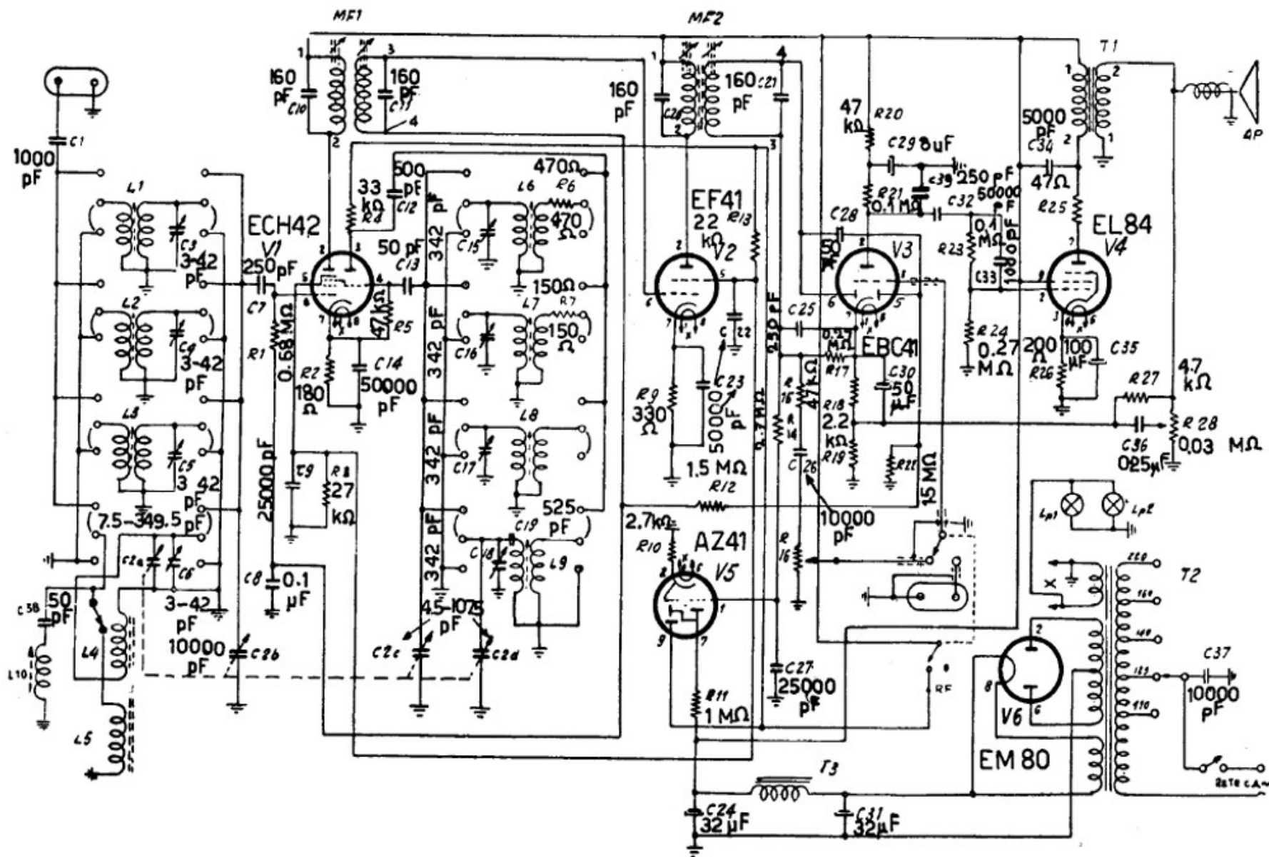
ALLOCCIO BACCHINI - Mod. 955/TA. Quattro gamme d'onda: una media e tre corte. Media frequenza 465 kc/s. Potenza di uscita 3,5 watt. Consumo 45 watt.
